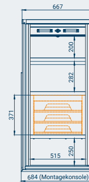
RoadBox RB-70 T: Ansicht Fahrerseite mit opt. Ladencontainer*
