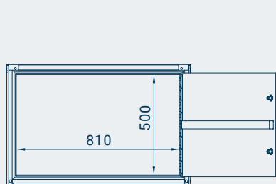
LongBox: Ansicht Beifahrerseite
