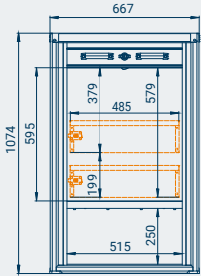
RoadBox RB-70: Ansicht Beifahrerseite mit opt. Auszugsladen*
