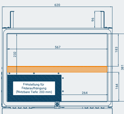
UnterflurBox UB-62: Beifahrerseite, mit Zwischenboden**
