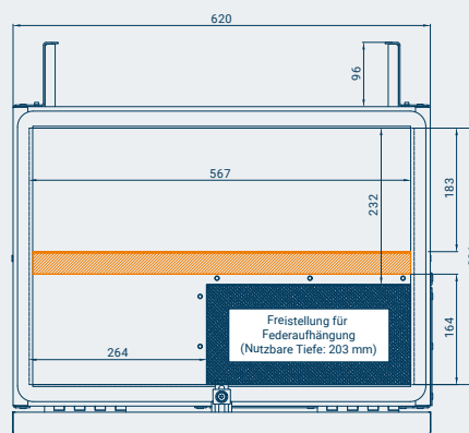
UnterflurBox UB-62: Fahrerseite, mit Zwischenboden**
