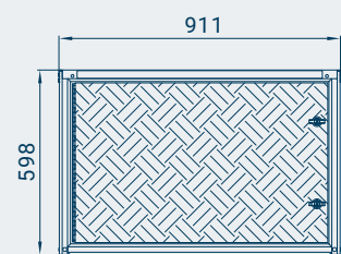
LongBox: Ansicht Fahrerseite
