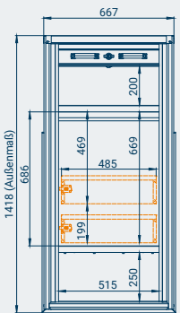
RoadBox RB-70 T: Ansicht Beifahrerseite mit opt. Auszugsladen*
