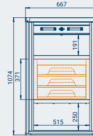
RoadBox RB-70: Ansicht Fahrerseite mit opt. Ladencontainer*
