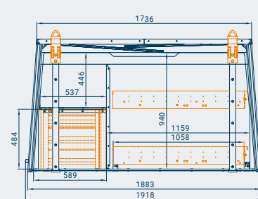
RB-125 / RB-150: Heckansicht mit optionalem Ladencontainer und Auszugsladen*
