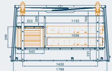
RB-125 / RB-150: Frontansicht mit optionalem Ladencontainer und Auszugsladen*
