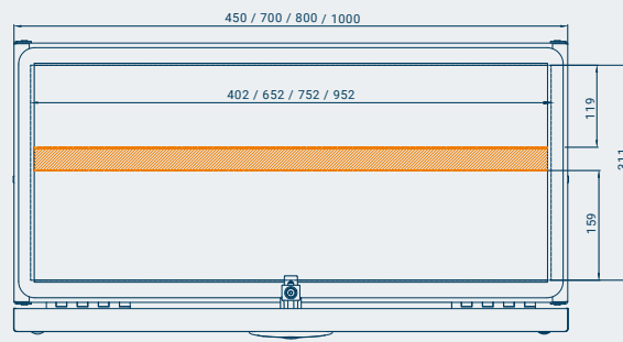
UnterflurBox UB-45 / UB-70 / UB-80 / UB-100: mit Zwischenboden**
