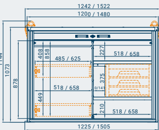
RB-125 / RB-150: Ansicht Beifahrerseite mit opt. Ladencontainer und Auszugsladen*
