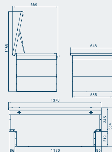
PickUp Box auf Ladefläche, in beladenem Zustand mit Fachteiler*
