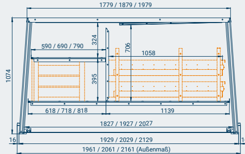
RoadBox RB-70: Heckansicht mit optionalem Ladencontainer und Auszugsladen*
