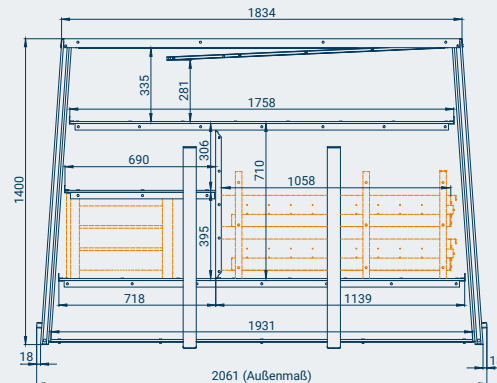
RoadBox RB-70 T: Heckansicht mit optionalem Ladencontainer und Auszugsladen*
