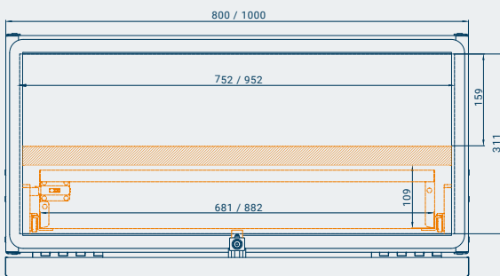
UnterflurBox UB-80 / UB-100: mit Auszugslade** und Zwischenboden**
