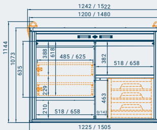
RB-125 / RB-150: Ansicht Fahrerseite mit opt. Ladencontainer und Auszugsladen*
